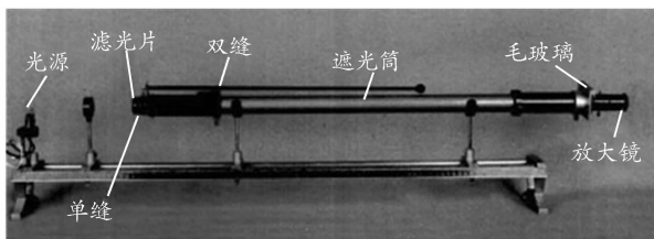
图1 双缝干涉的传统实验装置
