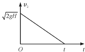
图4 v_2-t 图
